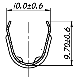
SECCION A-A
